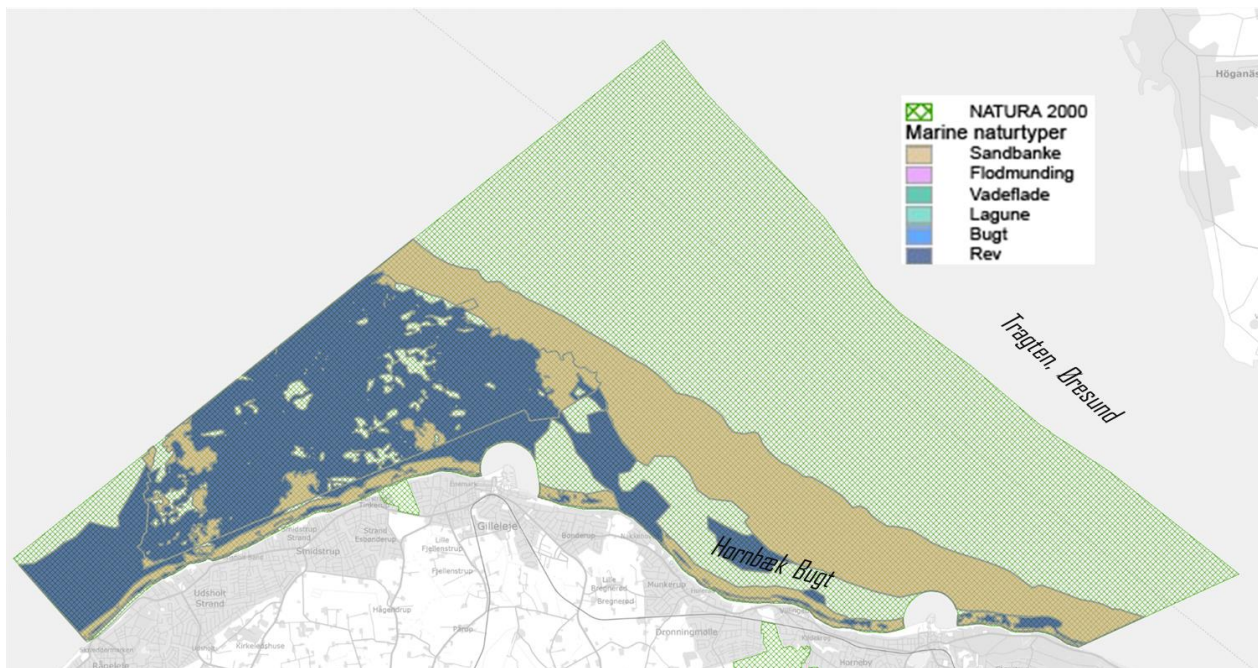
Figur 4. Det godt 150 km 2 store Natura 2000 område ud for Sjællands Nordkyst (Gilleleje Flak og Tragten), hvor også de beskyttede naturtyper er vist med sand i øst og stenede bundtyper i vest.
