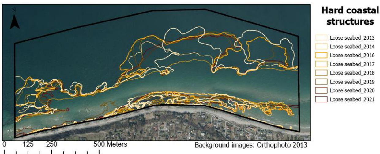
Figur 2. Kortlægning af områder med sandbund ved Gilbjerg Hoved 2013-2021. Analyse og kort ved specialestuderende Laura Strøm Magnér, IGN, KU
